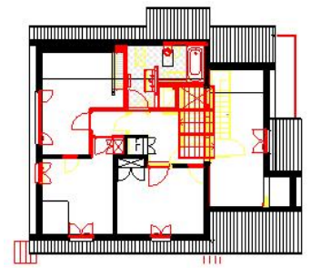
Dachgeschoss
